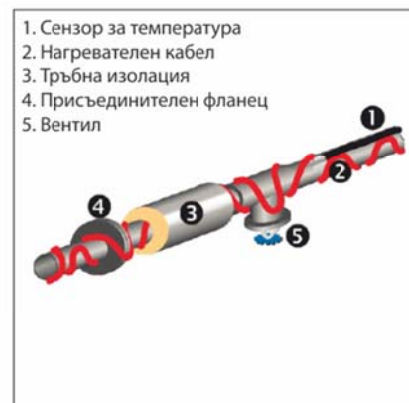
фиг. 4 Отопление на тръбна арматура
