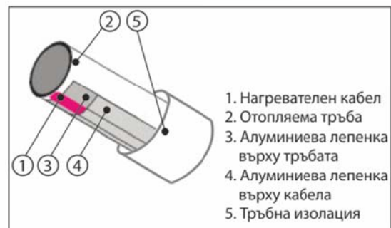
фиг.2 Отопление на PVC или PP тръба
