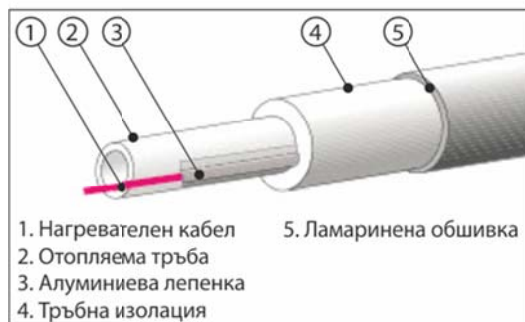
фиг.1 Отопление на метална тръба
