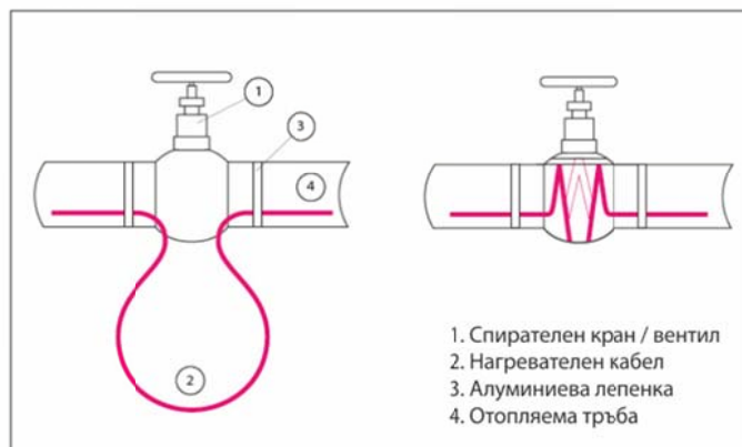
фиг. 3 Отопление на тръбна арматура
